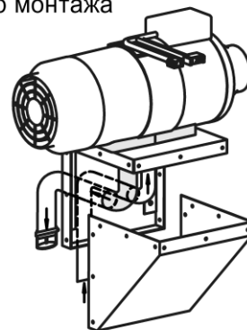
Защита выхлопной трубы и топливопровода
